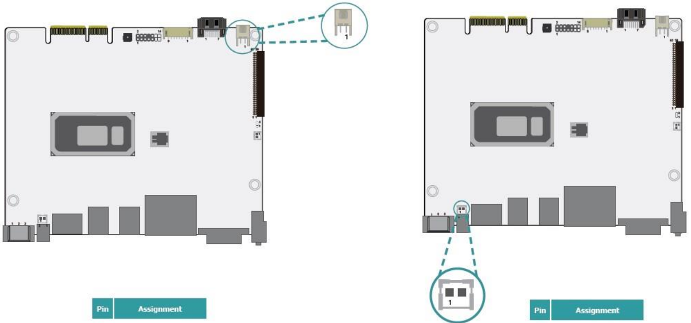
Reset Button (J44)
